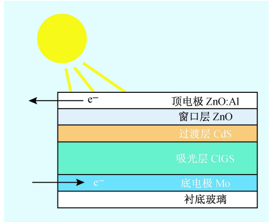
铜铟镓硒 \text{Cu}(\text{In}, \text{Ga})\text{Se}_2 , 简称 CIGS] 薄膜太阳能电池主要由底电极、P-N 结 CIGS/CdS 和顶电极三部分组成;太阳光透过透明导电的 \text{ZnO}:\text{Al} 层和 CdS 层,辐照到吸光层 CIGS 上激发出额外的电子-空穴对;在 P-N 结电场的作用下,额外产生的电子通过顶电极 \text{ZnO}:\text{Al} 层输往外电路,空穴则通过底电极 Mo 输往外电路,从而实现了光电转换
