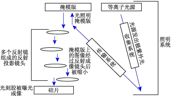
图 14 极紫外光刻机原理简图 Fig. 14 Schematic diagram of EUVL
